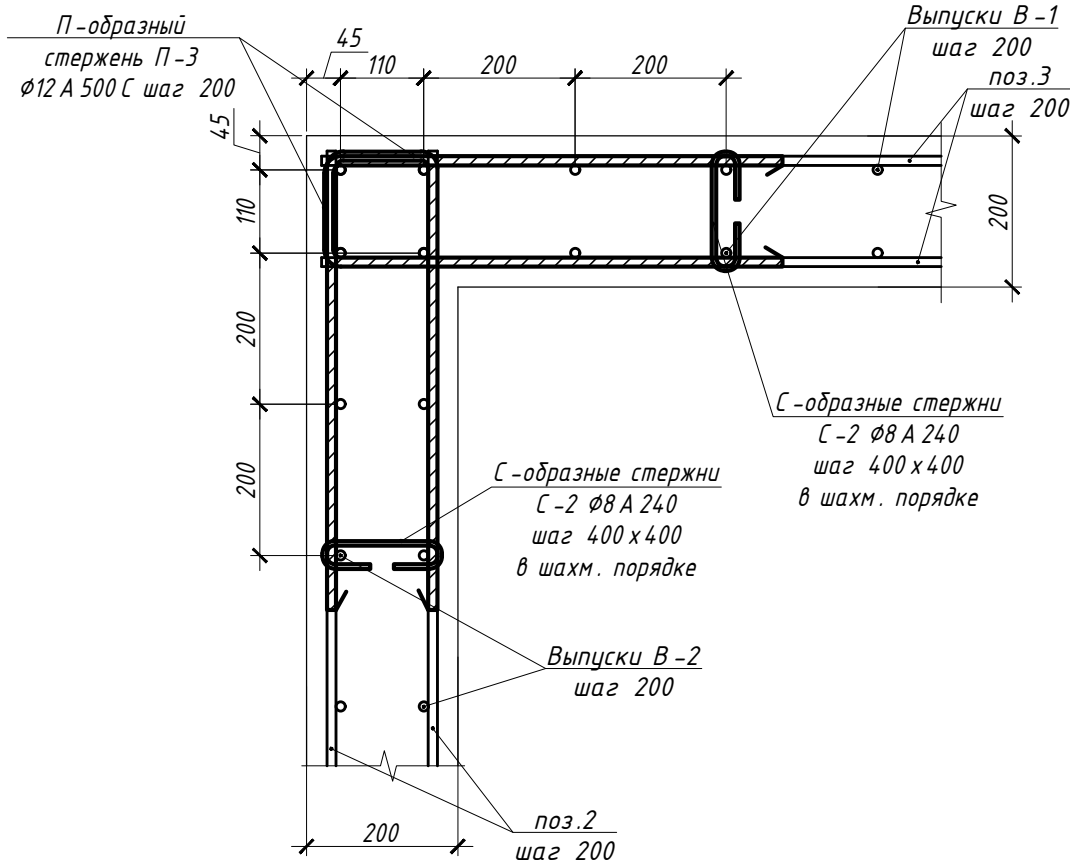
Узел 1 (М 1:10)
